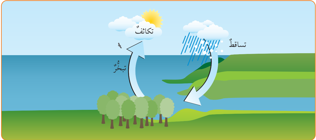
الشكل (8): كيفية حدوث الأمطار الحملية.
