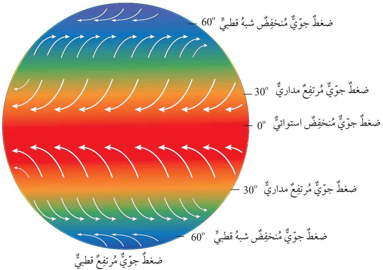
الشكل (3): نطاقات الضغط الجويّ الرئيسيّة في العالم.
