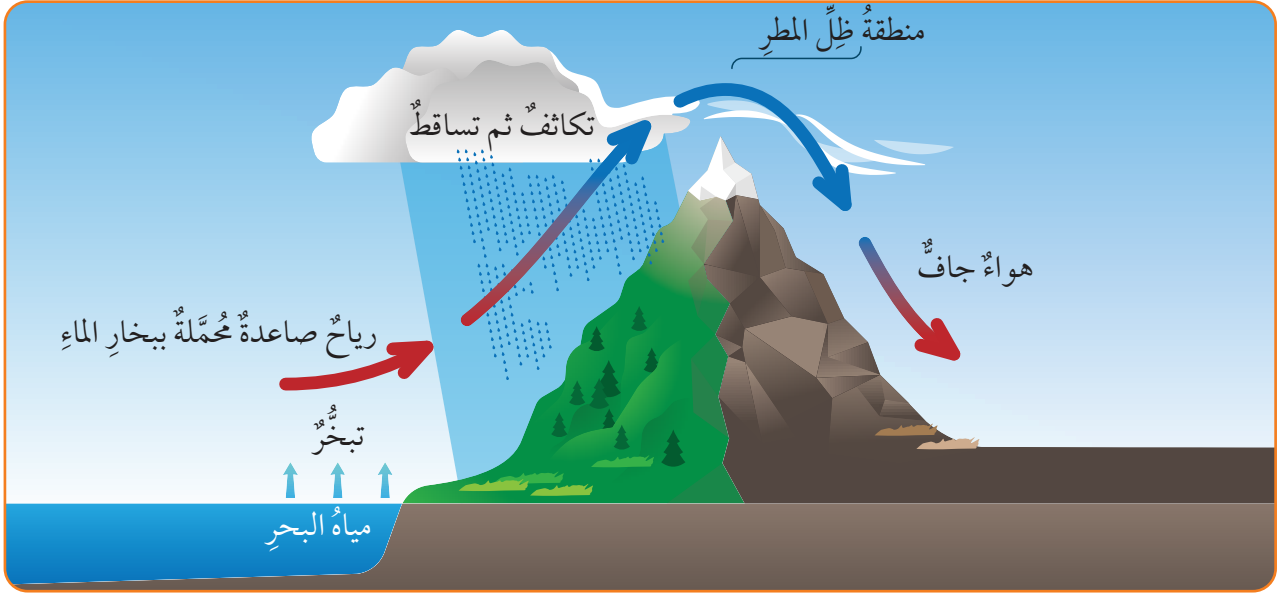
الشكل (7): كيفية حدوث الأمطار التضاريسية.
