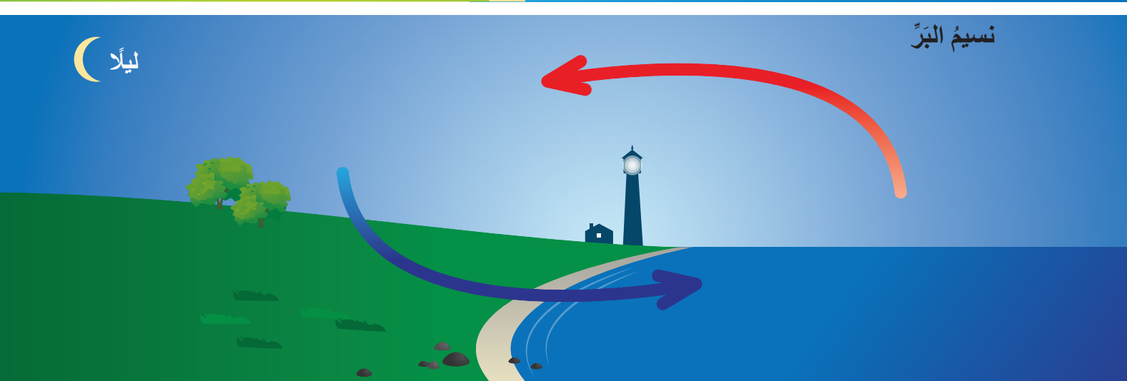
الشكل (5): آلية حدوثِ نسيمِ البرِّ ونسيمِ البحرِ.
