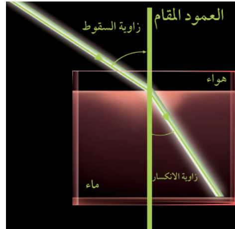
الشكل ٨ يحدث الانكسار عندما تغير الموجة سرعتها. وقد غيرت موجات الضوء اتجاهها، عندما نقصت سرعتها نتيجة انتقالها من الهواء إلى الماء.
