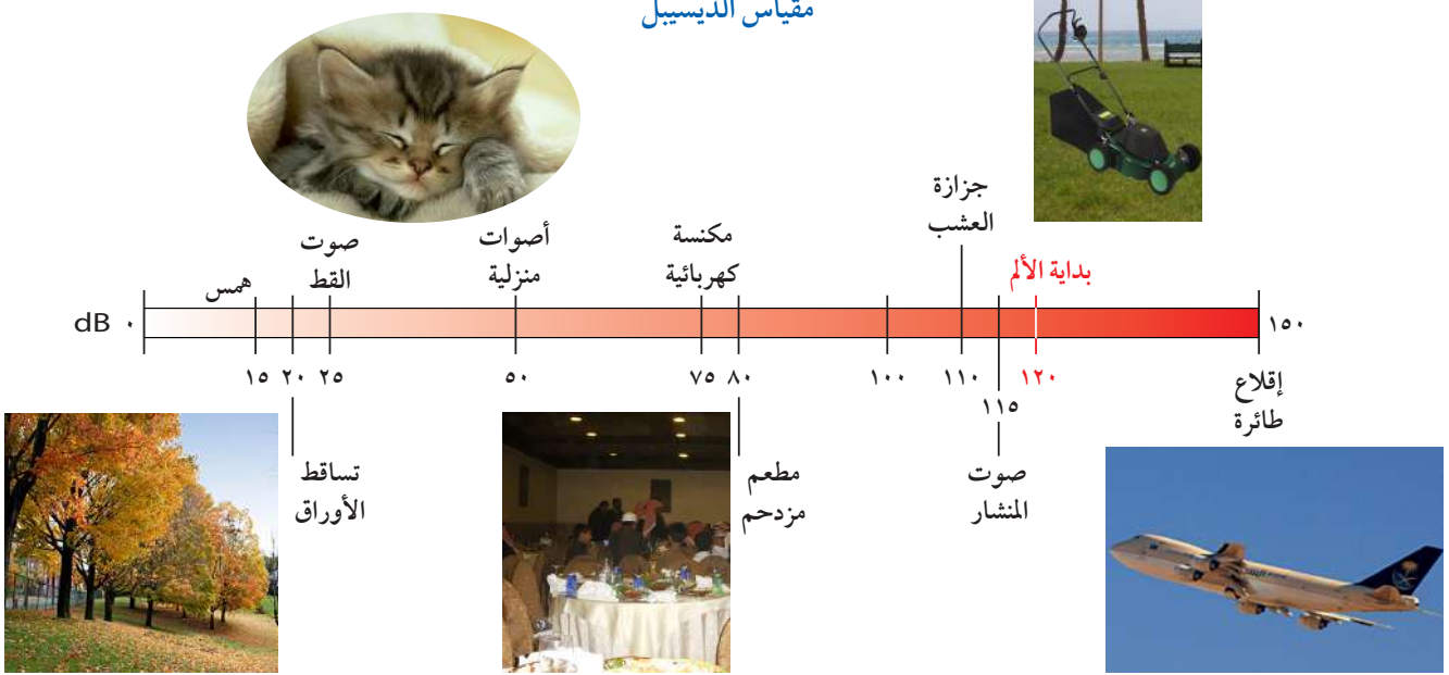
الشكل ١٣ يقاس مستوى شدة الصوت بوحدة ديسيبل.
