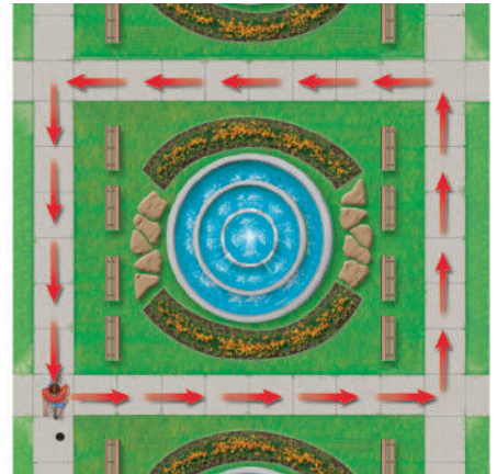
المسافة: ١٤٠ م الإزاحة: صفر
