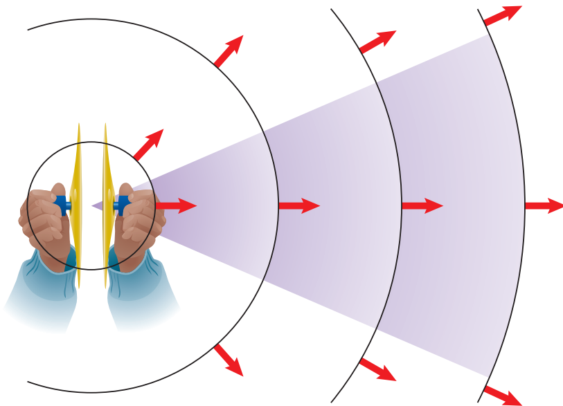
الشكل ١٢ تتناقص شدة موجات الصوت كلما انتشر الصوت مبتعداً عن مصدره؛ حيث تتوزع الطاقة التي تحملها موجات الصوت على مساحة أكبر.
