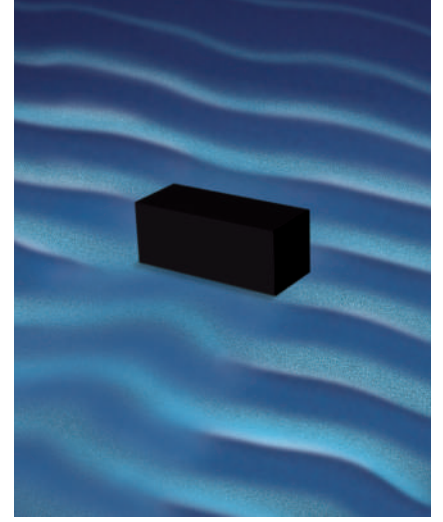
الشكل ٩ يعتمد حيود الموجة وانعطافها حول الجسم على حجم (أبعاد) الجسم وعلى طول الموجة.
