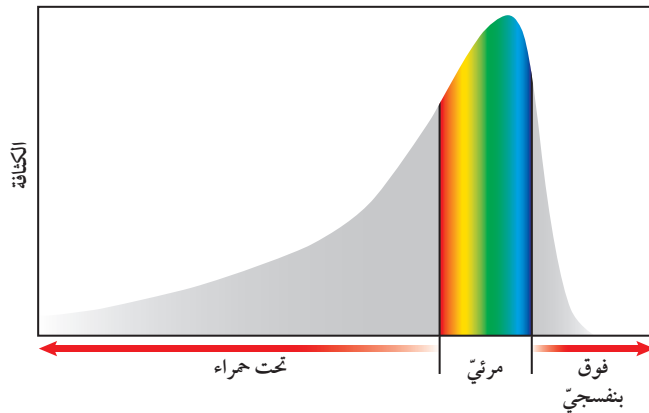
موجات كهرومغناطيسية من الشمس
