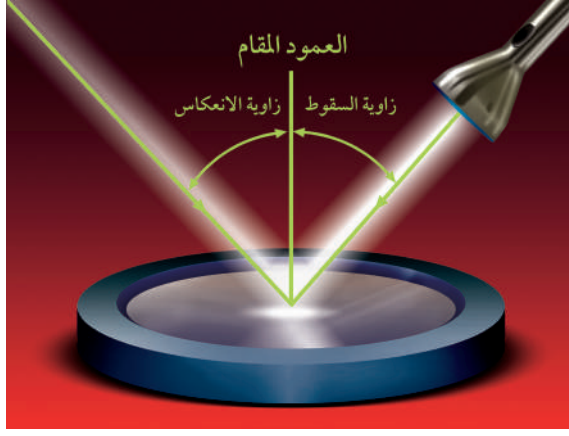
الشكل ٧ جميع الموجات تخضع لقانون الانعكاس، زاوية الانعكاس تساوي زاوية السقوط.
