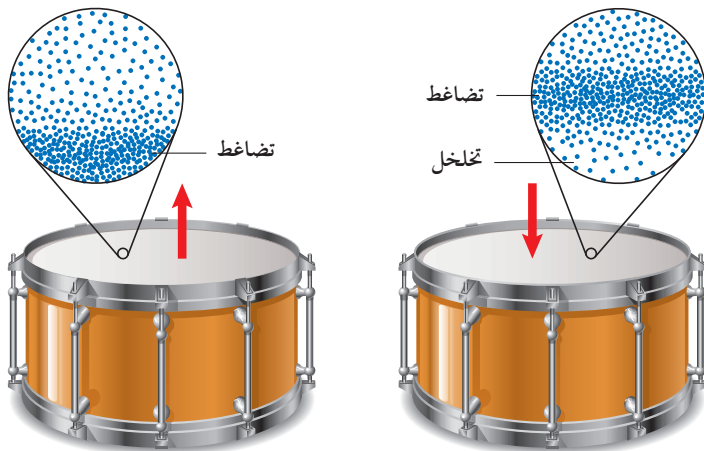
الشكل ١٠ اهتزاز غشاء الطبل يُنتج موجات صوتية؛ حيث يولد الغشاء تضاعطاً كلما اهتز نحو الخارج واخللاً كلما اهتز نحو الداخل.
