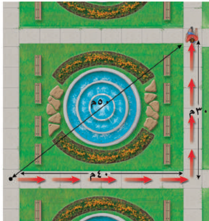
المسافة: ٧٠ م الإزاحة: ٥٠ م شمال الشرق
