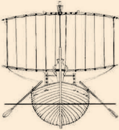
الشكل (١٥): مقطع هندسيّ للسفينة ذاتها.
