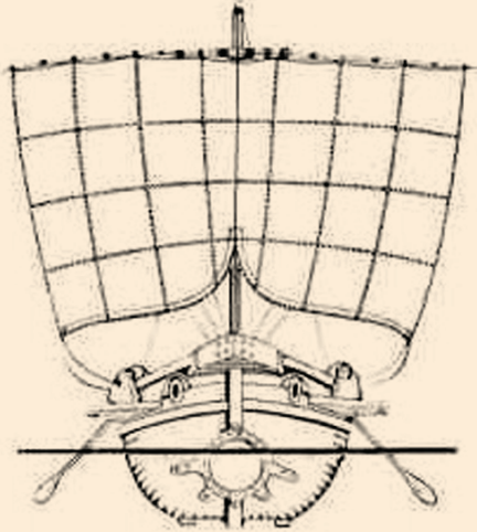
الشكل (١٧): مقطع هندسيّ للسفينة ذاتها.
