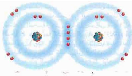
الرابطية الثنائية
