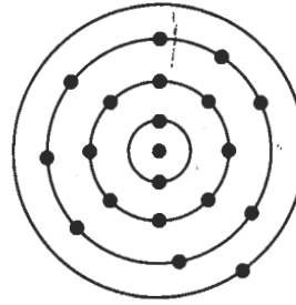
K العدد الذري 19
