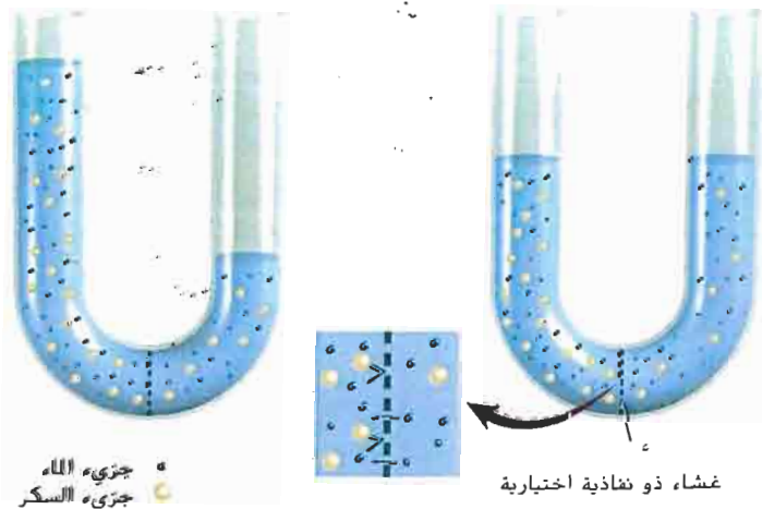
بعد الأسموزية
