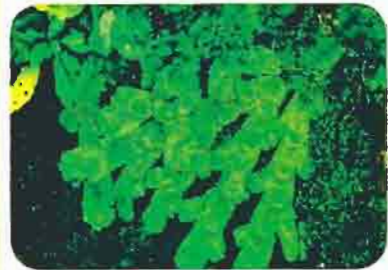
نباتات كبدية
