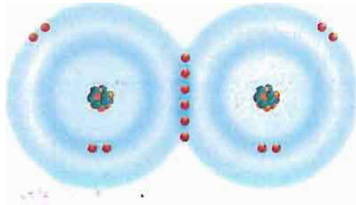
الرابطية الثلاثية
