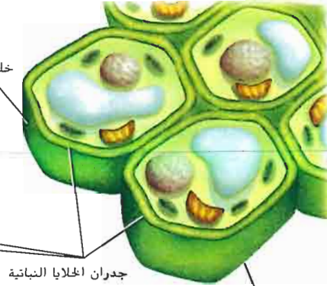
خلية نباتية 1
