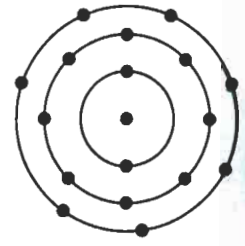
Cl العدد الذري 17
