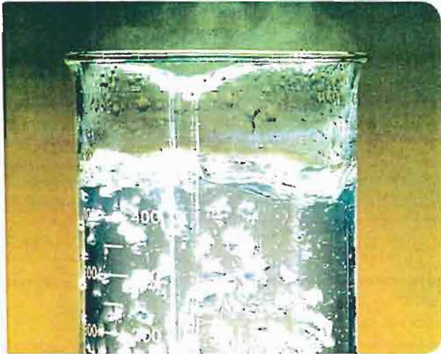
تغير فيزيائي
