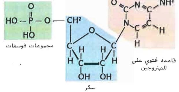
نيوكليوتيد
