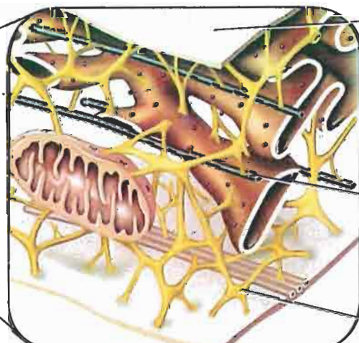
الهيكل الخلوي
