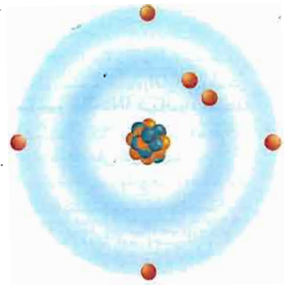
الكربون
