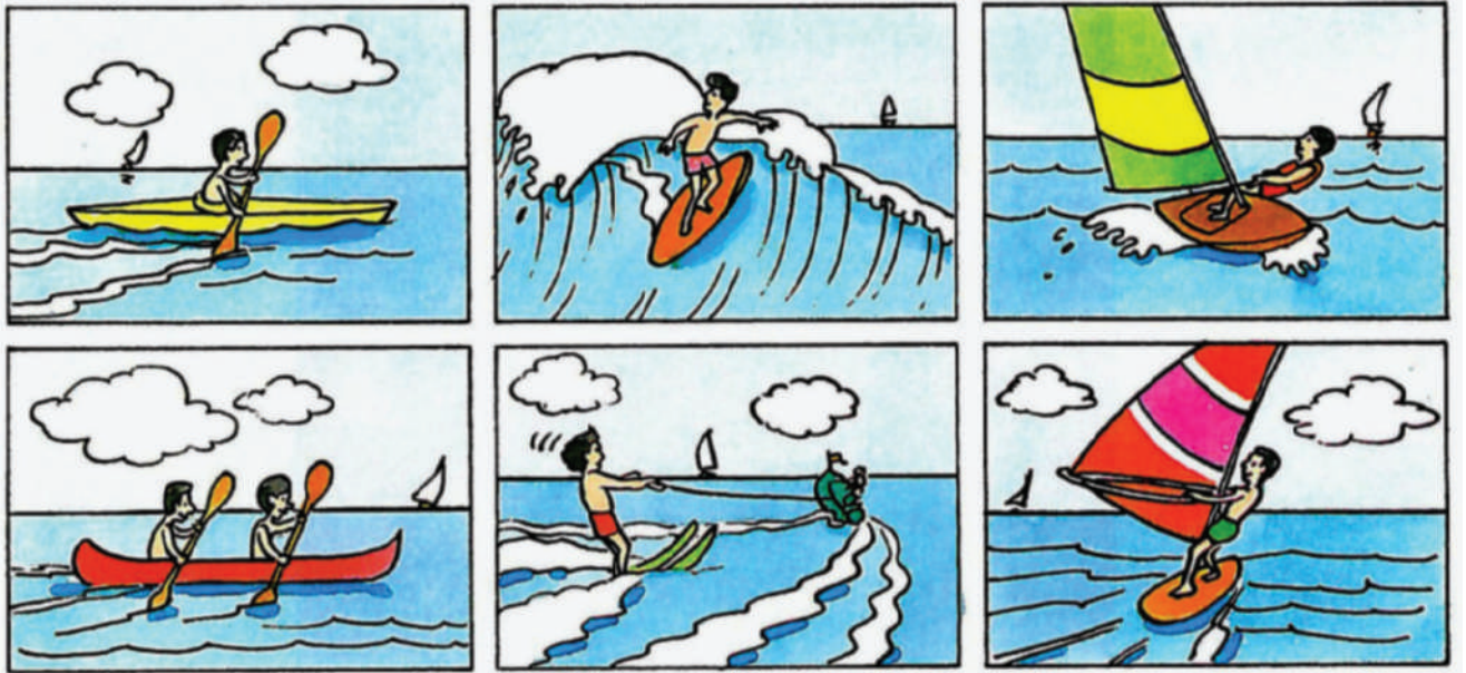
٧- رياضات بحرية
