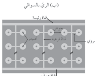
الشكل (١-٤٧): أنظمة الري المستخدمة في حقول النخيل.
