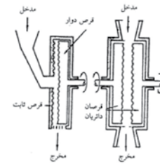
الشكل (١-٣٦): أقراص الجرش.
