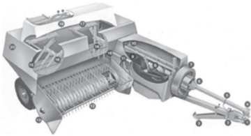
الشكل (٢٩-١): أجزاء مكابس البالات المستطيلة المقطع.
