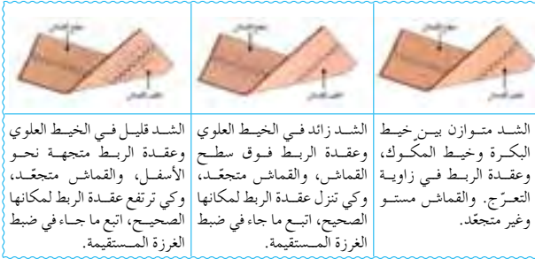
الشكل (٢-٣٨): ضبط الشد في الغرزة المتعرجة.
