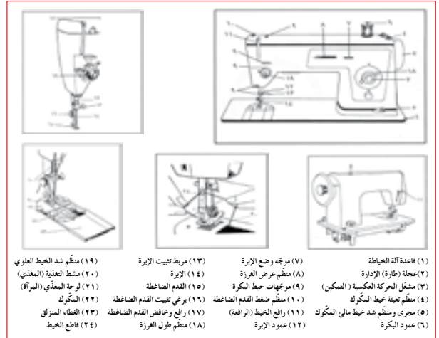
الشكل (٢-٤): أجزاء آلة الخياطة المنزلية.
