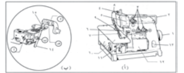
الشكل (٢-٥): أجزاء آلة الحبكة ذات الخيوط الثلاثة.
