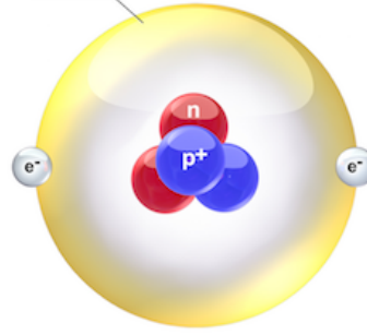
ذرة الهيليوم
